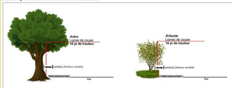
Gabarit pour taille d'arbres et d'arbustes
