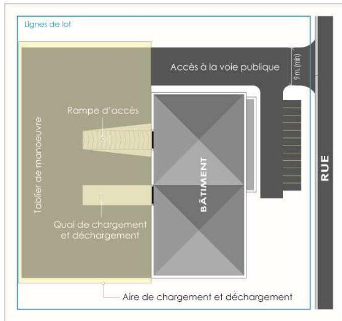
Illustration 23 Aire de chargement et déchargement
