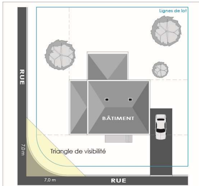
Illustration 14 Triangle de visibilité
